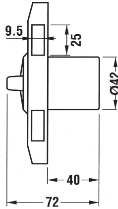
Thumbturn
